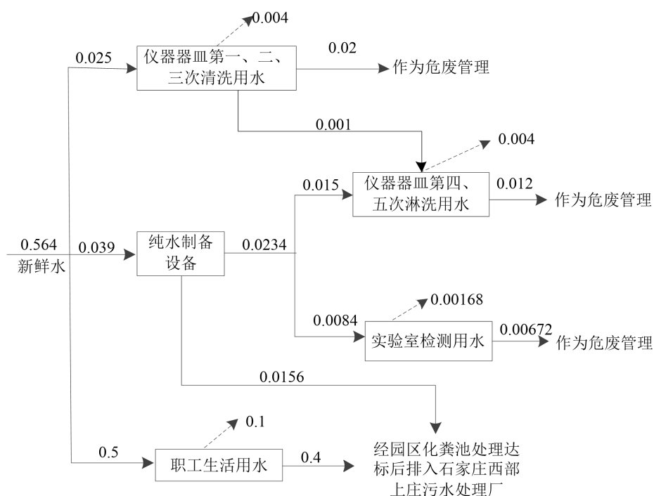
图 2-1 项目水量平衡图 单位 \text{m}^3/\text{d}
