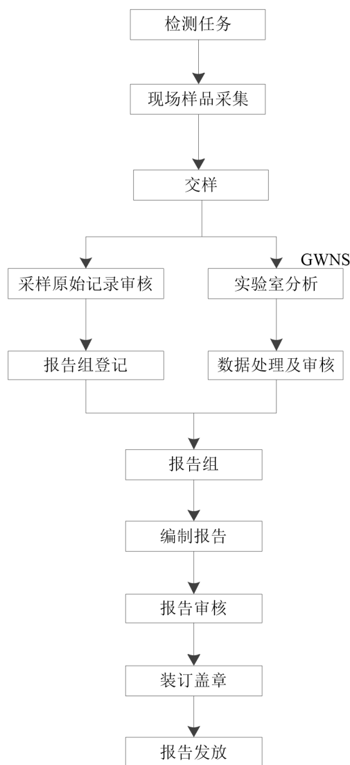
图 2-2 检验流程图及排污节点图
