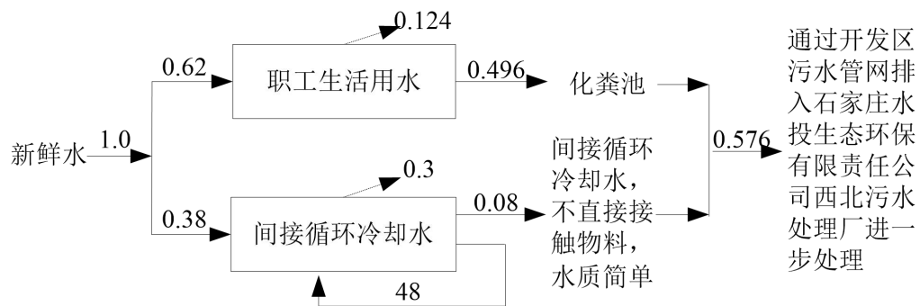
图3 本项目给排水平衡图
