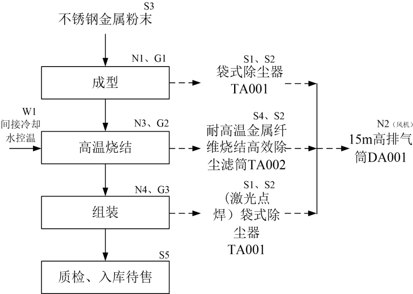
图4 本项目生产工艺流程图 表19 本项目排污节点一览表
