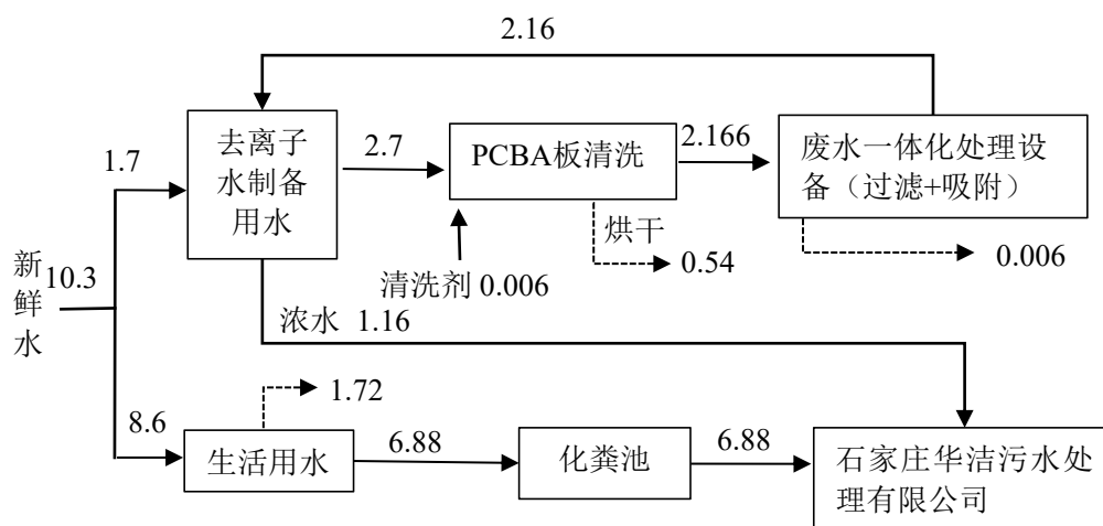
图 2-2 全厂给排水平衡图 单位：m³/d
