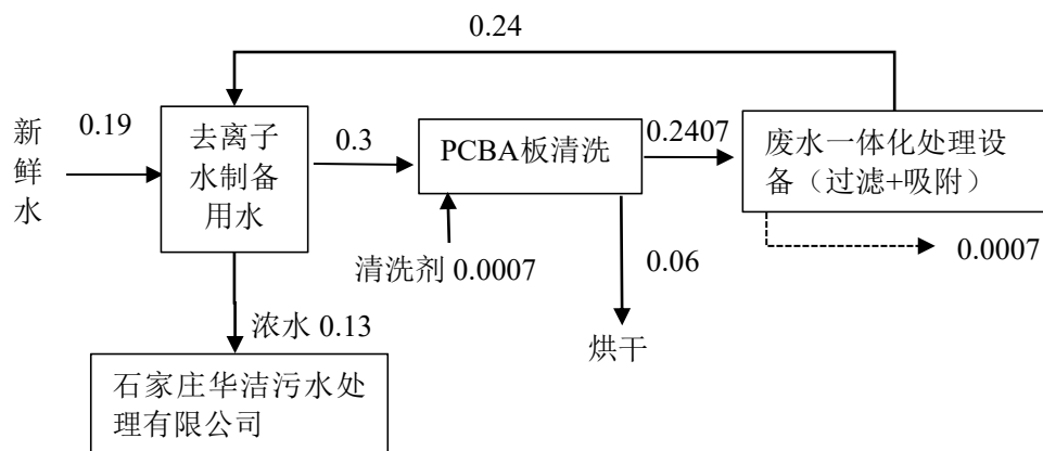
图 2-1 本项目水平衡图 单位：m³/d
