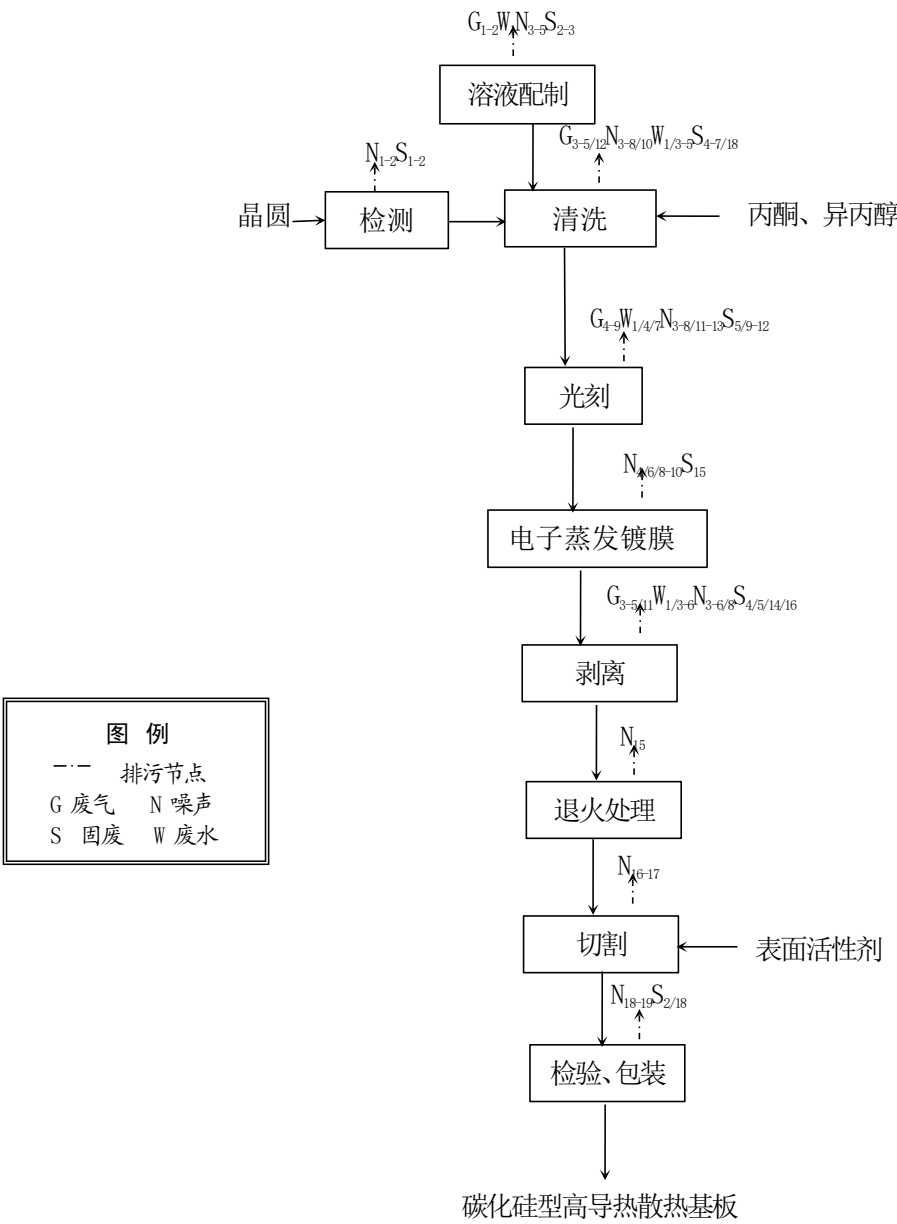
图 2-3 本项目碳化硅型高导热散热基板生产工艺流程及排污节点图
